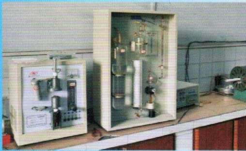
定碳分析装置
